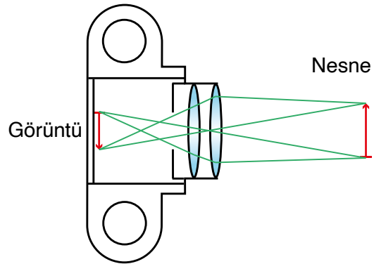
▲ Görsel 1.5.2: Kamerada görüntü oluşumu
