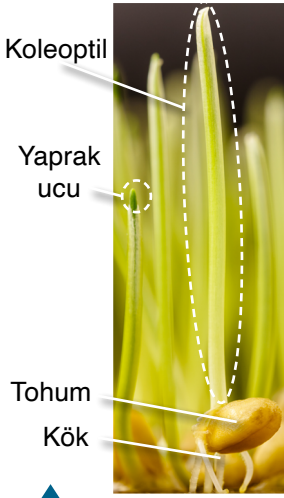
Görsel 1.4.2: Koleoptil
